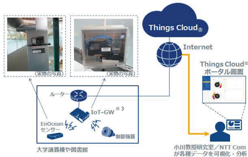
(図：実証実験の構成図←クリックして拡大)
