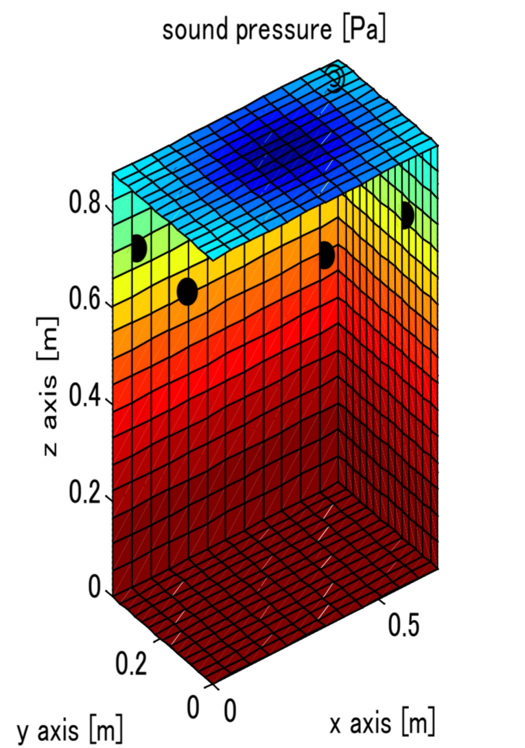
(A) 制御前
