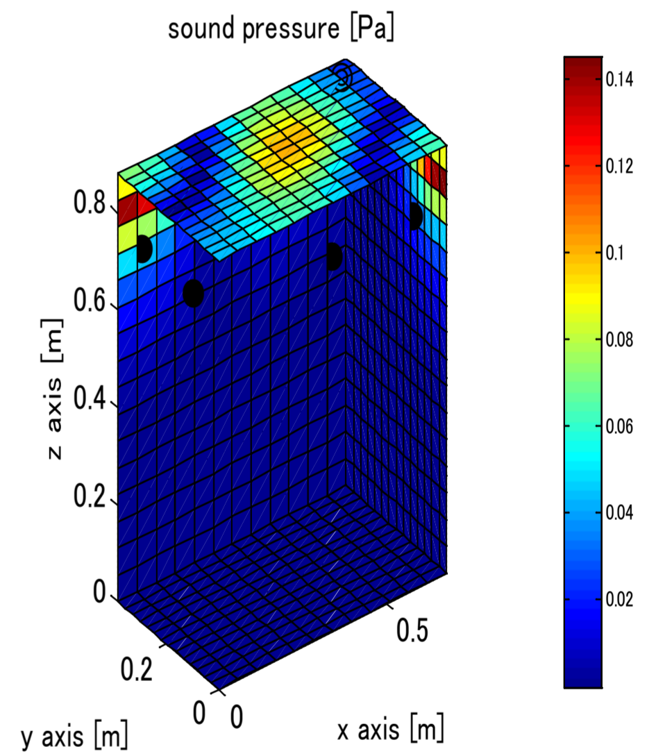
(B) 制御後
